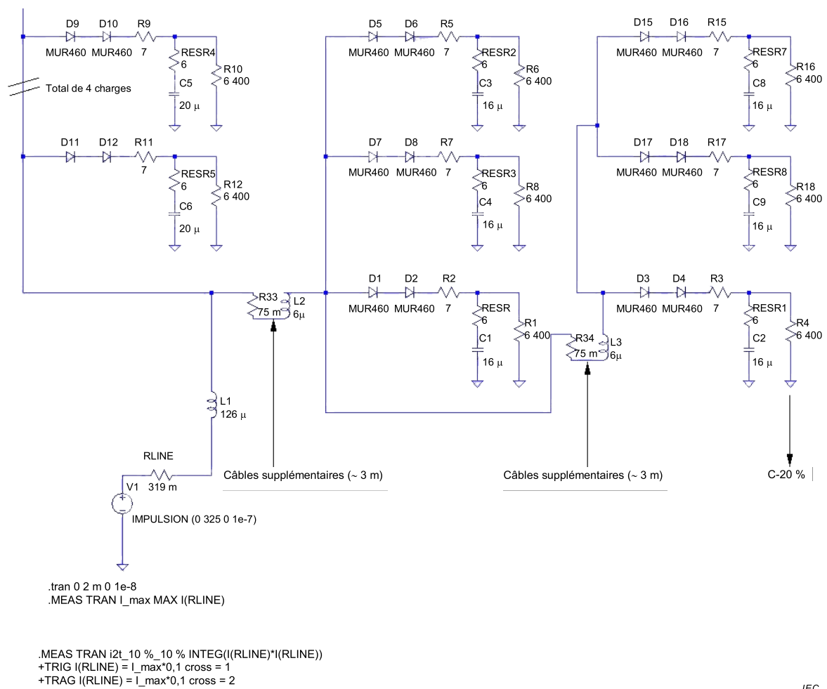
Figure C.3 – Modèles pour charges de lampes multiples
