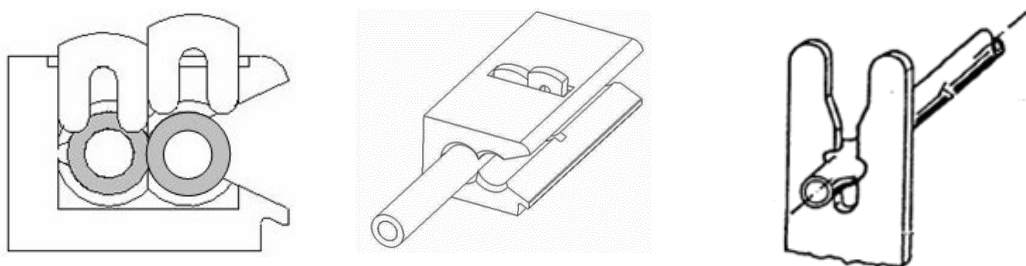
Figure D.1 – Exemple de bornes à perçage d'isolant
