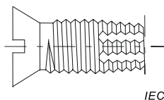
Figure 7 – Vis autotaraudeuse à découpe de matière
