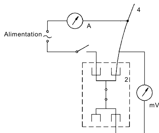
Figure 10b – Exemple de disposition d'essai pour le mesurage de la chute de tension lors de l'essai de déflexion sur les bornes sans vis
