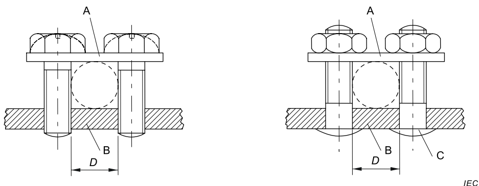
Figure 2 – Bornes à serrage sous tête de vis et bornes à goujon fileté
