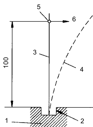
Figure 10a – Principe de l'appareil d'essai pour les essais de déflexion sur les bornes sans vis
