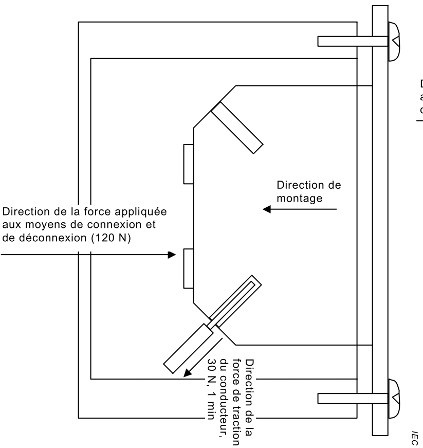
Figure 22a – Détermination de la direction des forces à appliquer
