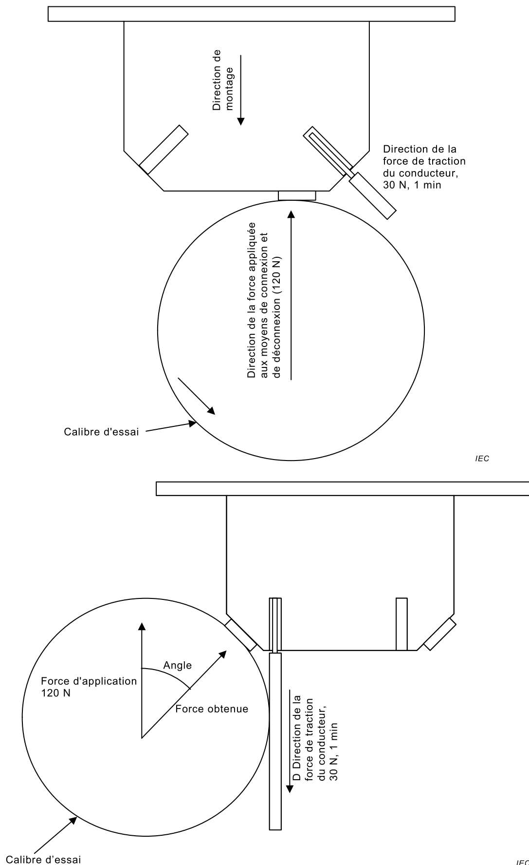
Figure 22b – Montage d'essai
