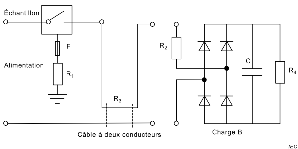
Figure 12b – Schémas de circuit pour l'essai des interrupteurs conformément à 19.3
