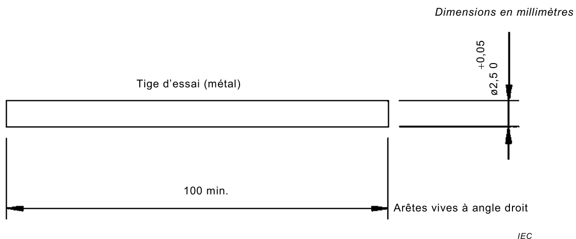
Figure 17 – Calibre de vérification des rainures, trous et conicités inverses
