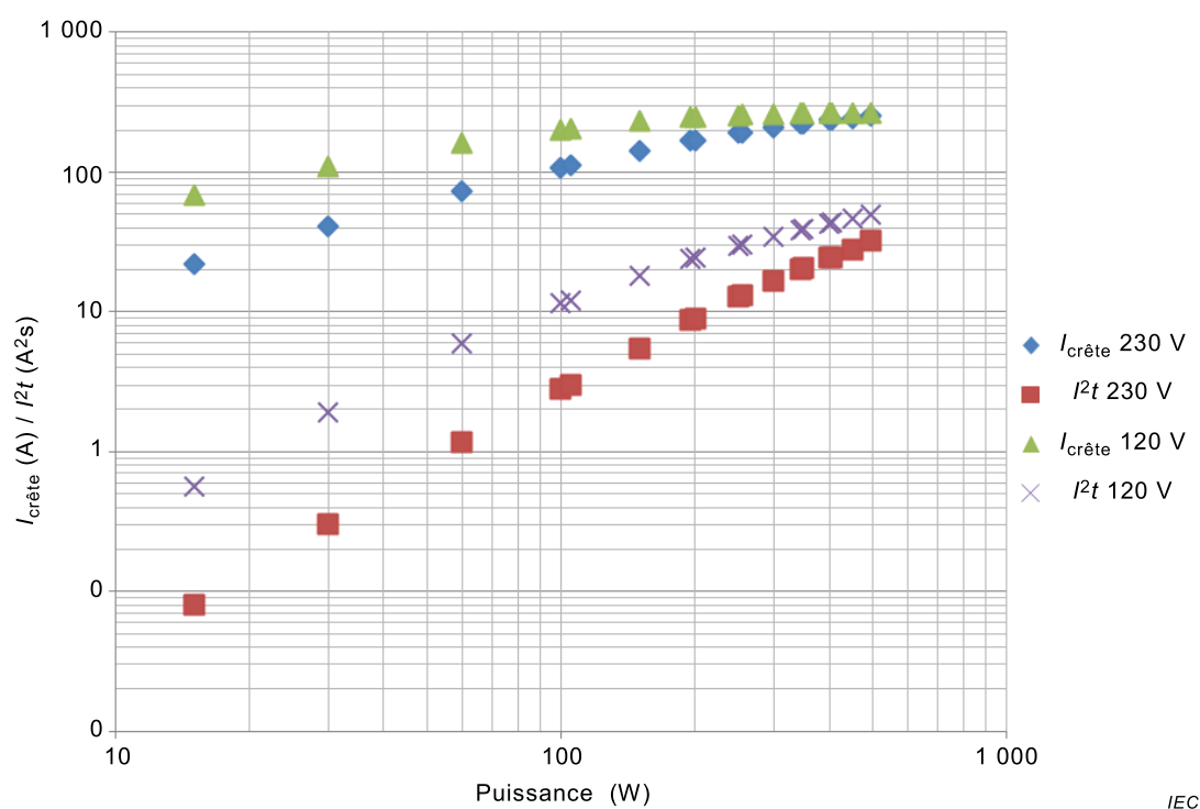
Figure C.4 – I_{\text{crête}} et I^2t pour charges de lampes multiples
