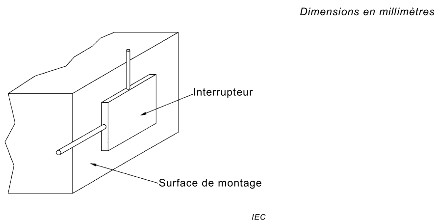
Figure 18 – Croquis indiquant la direction d'application du calibre de la Figure 17
