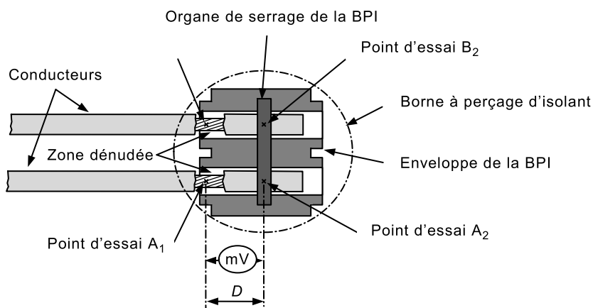
Figure D.1 – Exemple de bornes à perçage d'isolant
