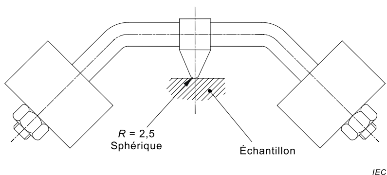
Figure 19 – Appareil pour l'essai à la bille
