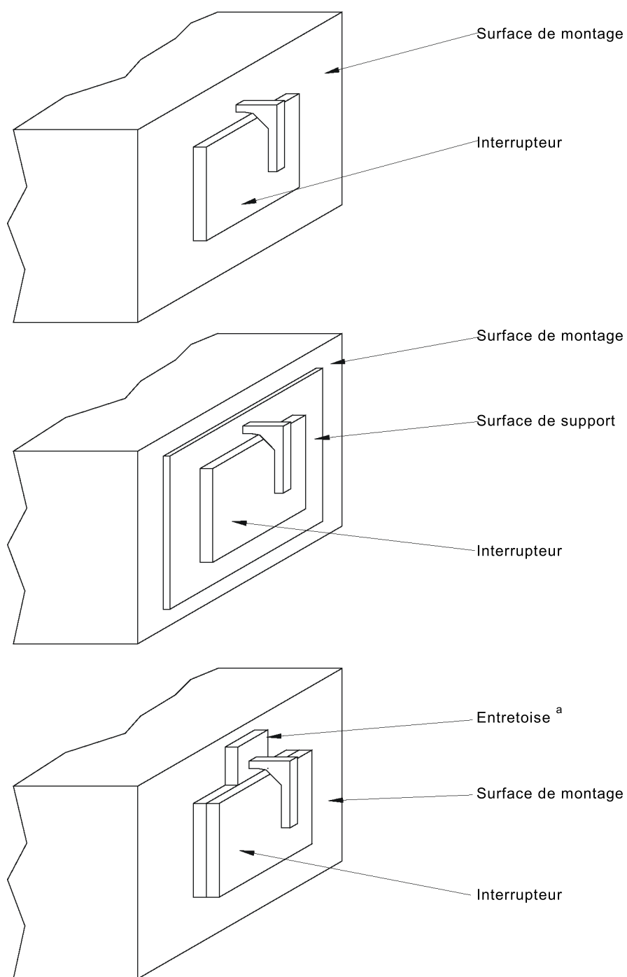
Figure 15 – Exemples de l'application du calibre de la Figure 14 sur des capots fixés sans vis sur une surface de montage ou de support
