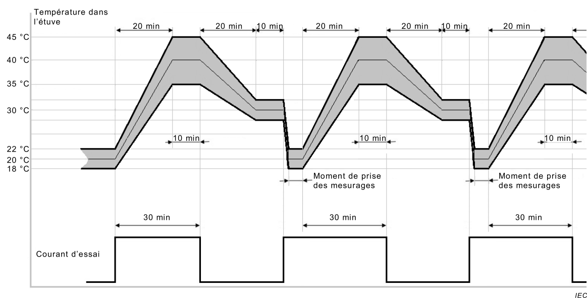
Figure D.3 – Cycle de température pour l'essai de chute de tension de 12.4.11
