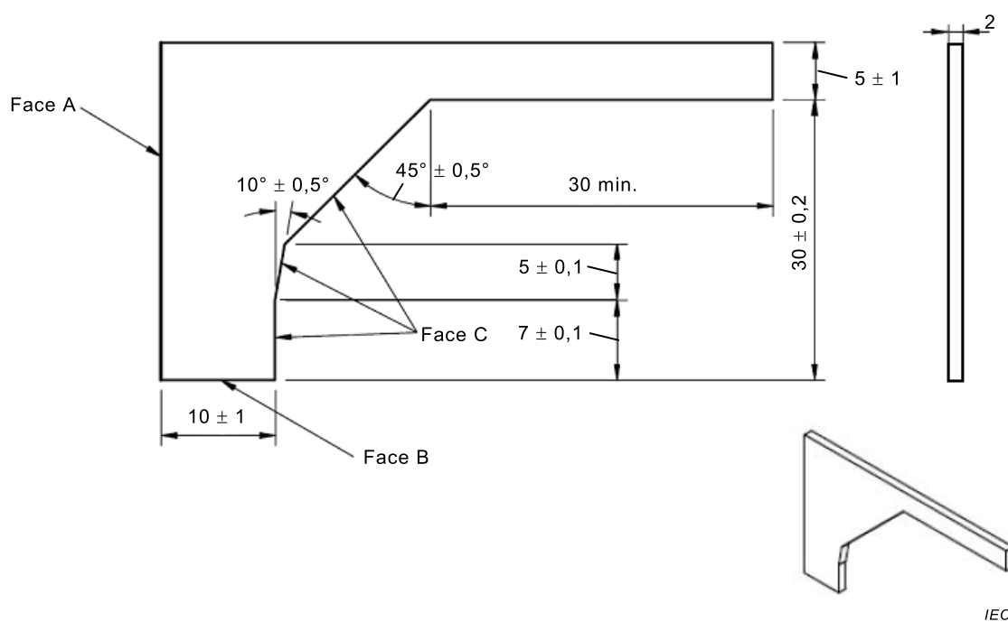
Figure 14 – Calibre (épaisseur: environ 2 mm) pour la vérification du contour des capots, plaques de recouvrement et organes de manœuvre
