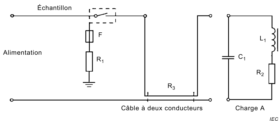
Figure 12a – Schémas de circuit pour l'essai des interrupteurs utilisés avec des charges par lampes à ballast externe
