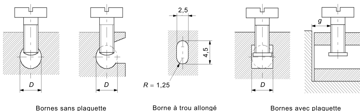
Figure 1 – Bornes à trou
