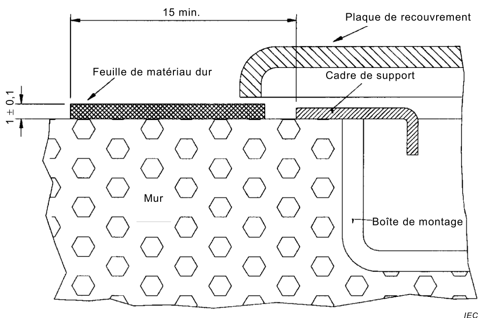
Figure 13 – Disposition pour l'essai des plaques de recouvrement
